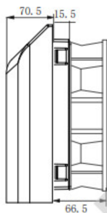
风扇过滤器 Fan filter
