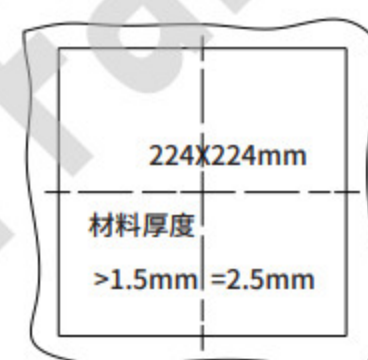
安装尺寸 Mounting dimension
