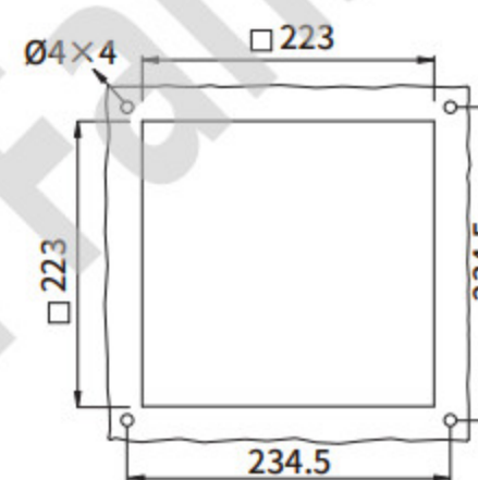
安装尺寸 Mounting dimension
