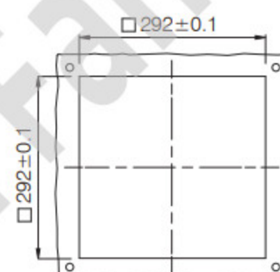
安装尺寸 Mounting dimension
