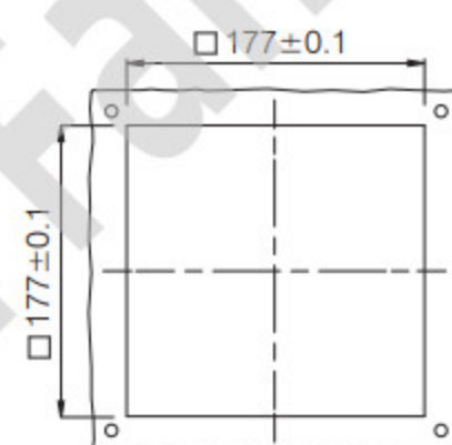
安装尺寸 Mounting dimension
