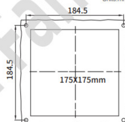
安装尺寸 Mounting dimension
