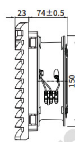
风扇过滤器 Fan filter
