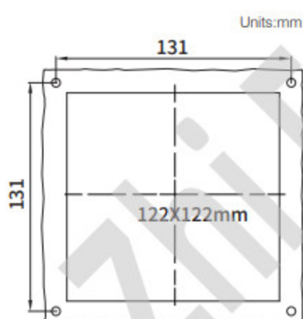
安装尺寸 Mounting dimension
