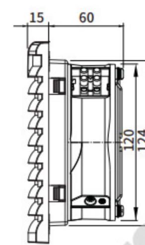
风扇过滤器 Fan filter
