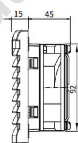
风扇过滤器 Fan filter
