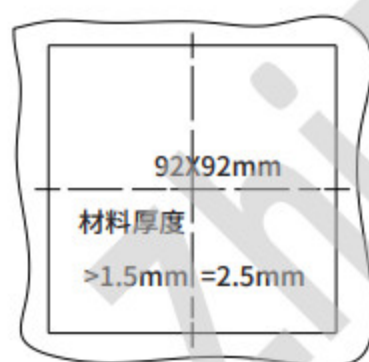
安装尺寸 Mounting dimension
