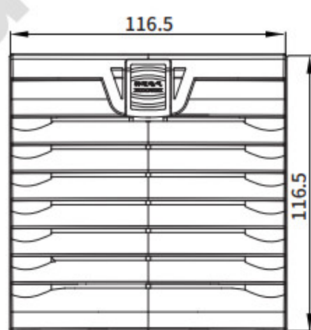
风扇过滤器 Fan filter
