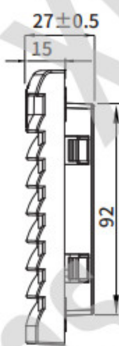
排气过滤器 Outlet filter
