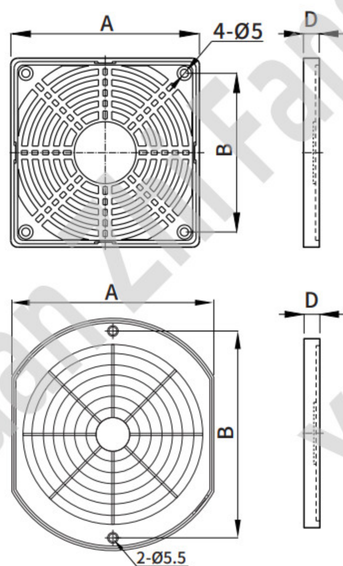
尺寸图 Dimension drawing
